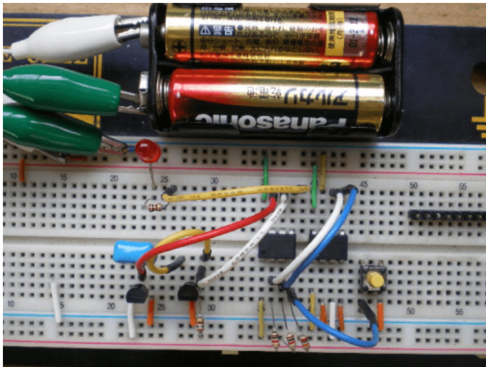
左側からLED、LM60、TL431、PIC12F683、24LC1025、スイッチの順です。
