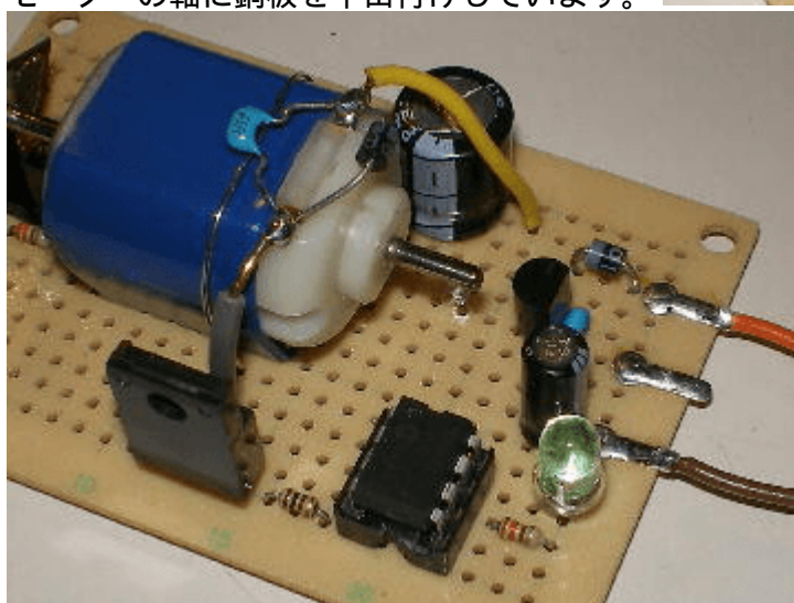
モーターの軸に銅板を半田付けしています。
