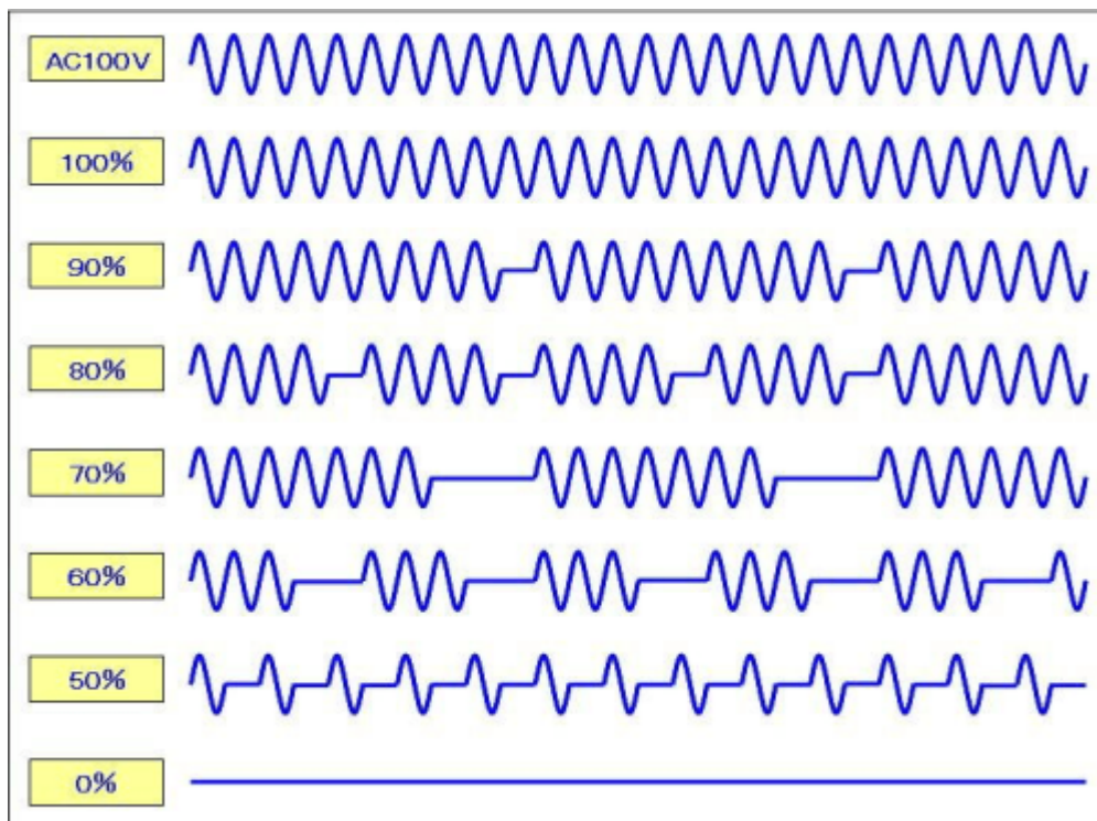
出力波形
