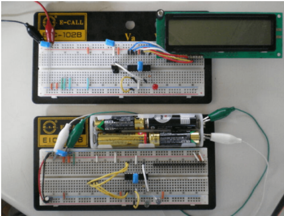
左側:受信モード時の回路です。 右側:送信モード時の回路です。
