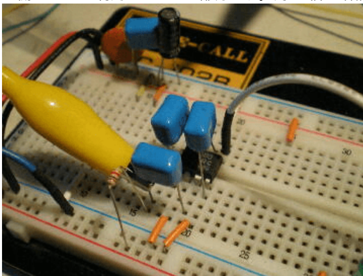
左側:LM386を利用したアンプ部分です。約200倍の増幅率があります。 右側:PIC16F88周りです。
