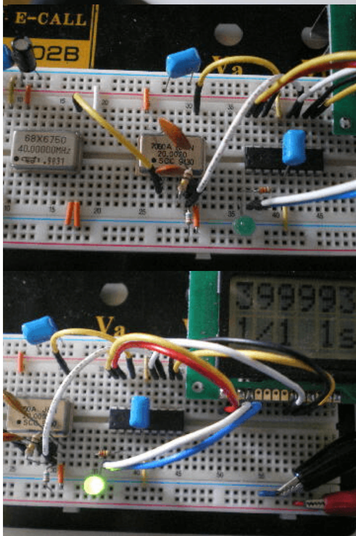
20MHzを測定しました。(プリスケアラ無し、ゲートタイム1秒)
